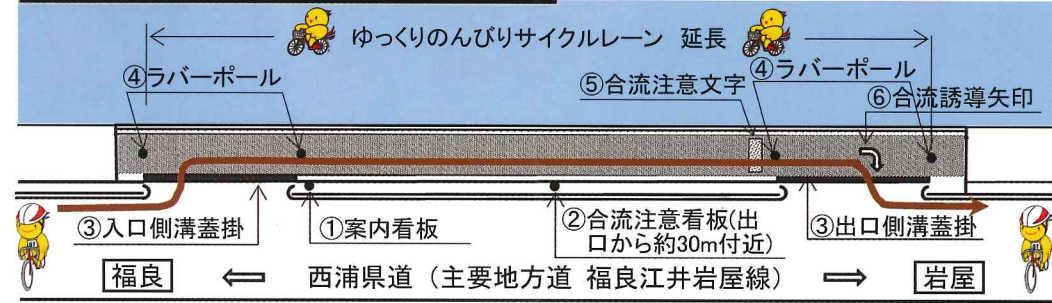
「ゆっくりのんびりサイクルレーン」概略図
